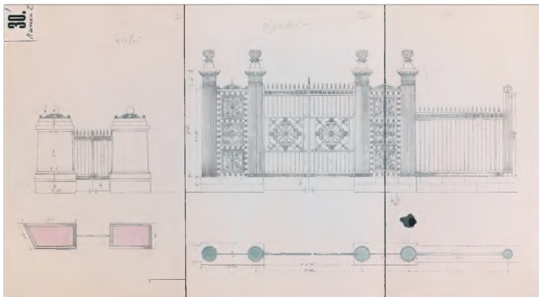
10. Фасад и план Грота в Кремлевском (Александровском) саду. Чертеж. Вторая половина XIX в. ОРПГФ Музеев Московского Кремля
