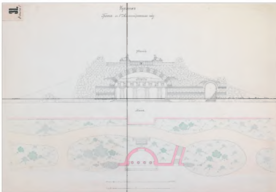
9. Фасад и план Грота в Первом Александровском саду. Чертеж. ОРПГФ Музеев Московского Кремля
